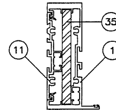
JAMB 'J4'
