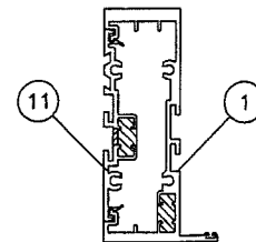
JAMB 'J3'
