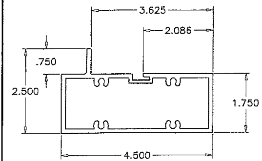
FRAME TRANSOM
