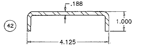
DOOR STOP
