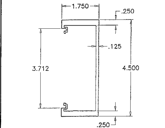
FRAME JAMB
