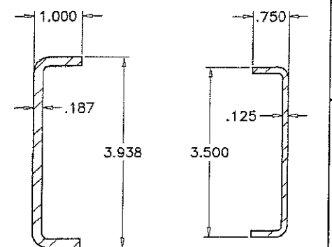
ASTRAGAL STILE
