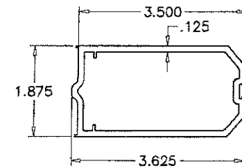
8A ALT. DOOR STILE
