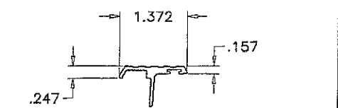
ASTRAGAL STILE
