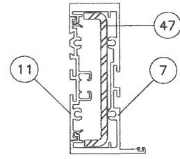
JAMB 'J2A'
